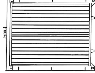
SECTION D-D 1:10
